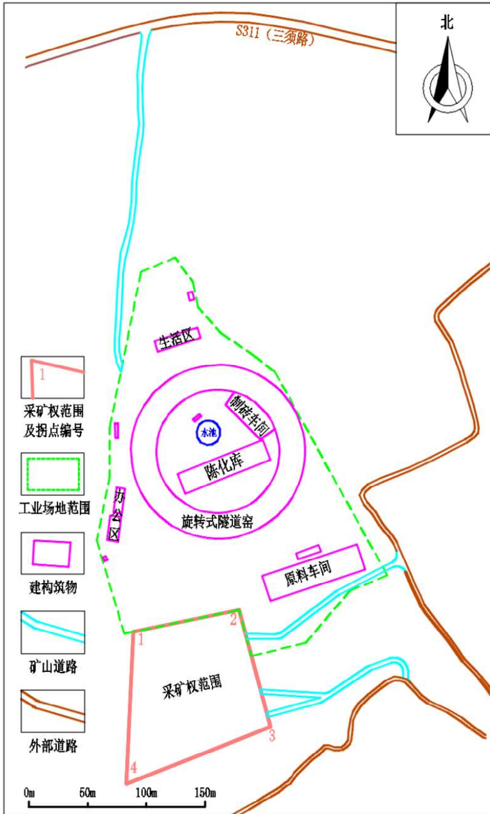
图 1-1 矿山总平面布置图
